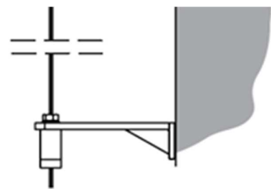
Spannwinkel mit Fassadenspanner
